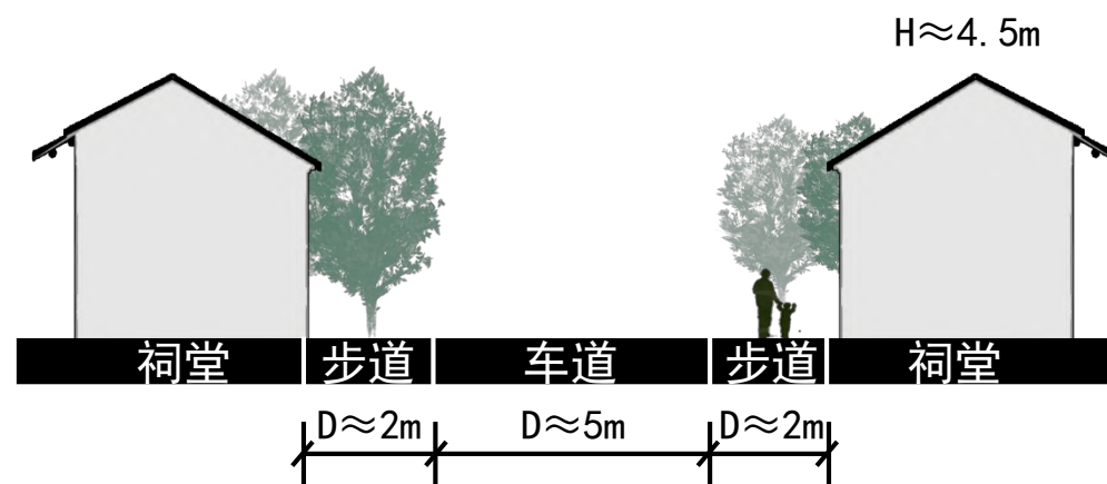
沙水路 高宽比 H/D \approx 0.5
