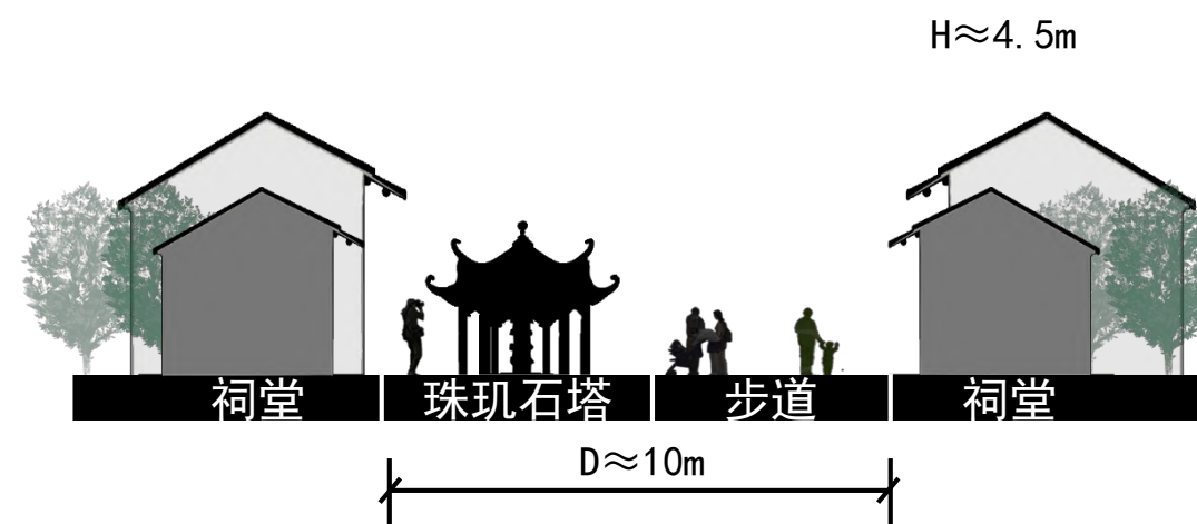
珠玑街最宽处 高宽比 H/D \approx 0.45
