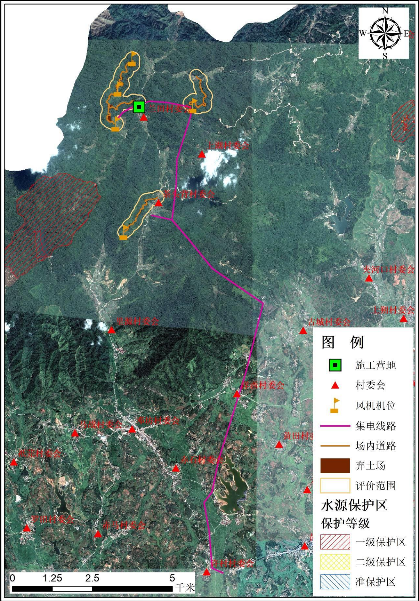
附图 3 项目与水源保护区位置关系图
