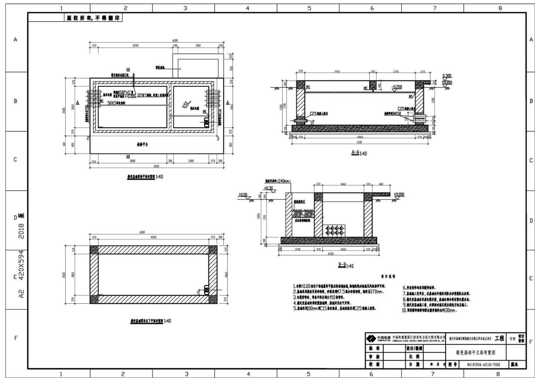
附图 12 箱变基础结构图
