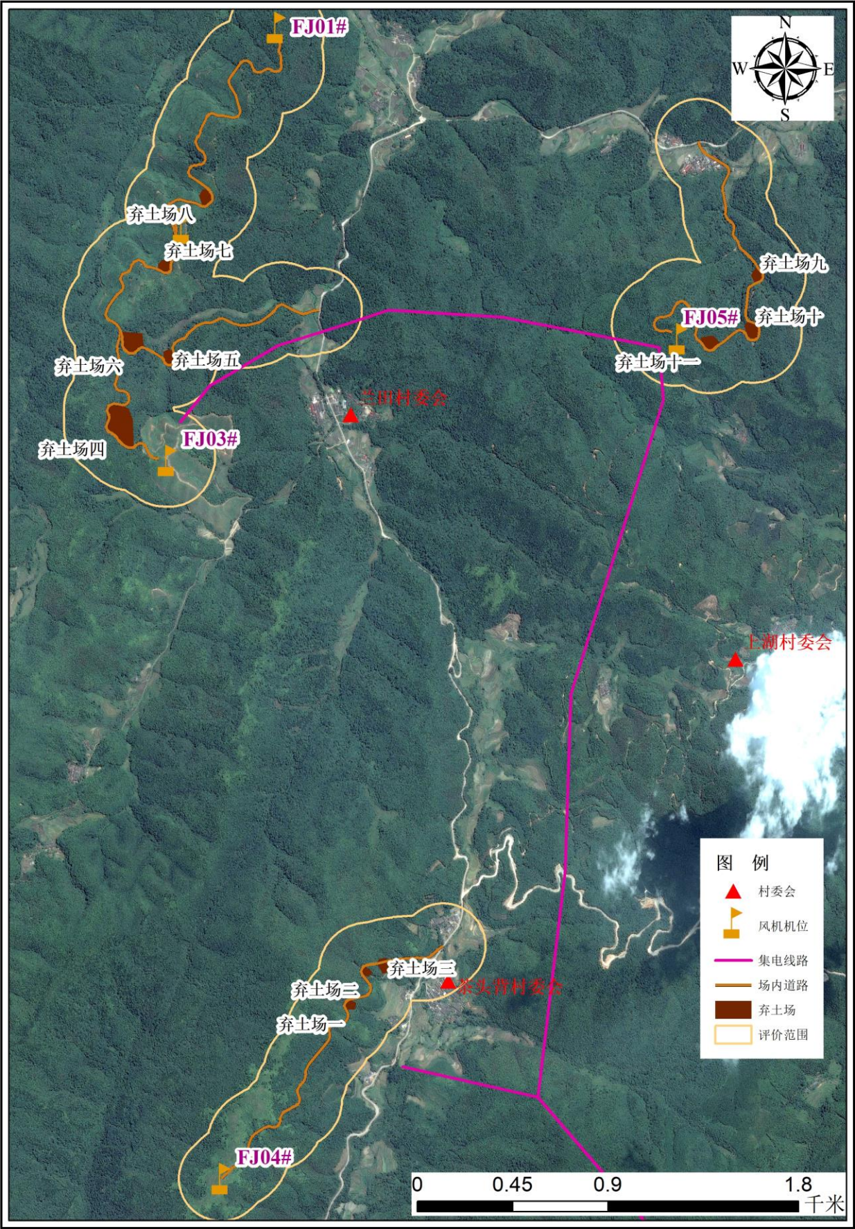
附图 19 项目弃土场分布示意图
