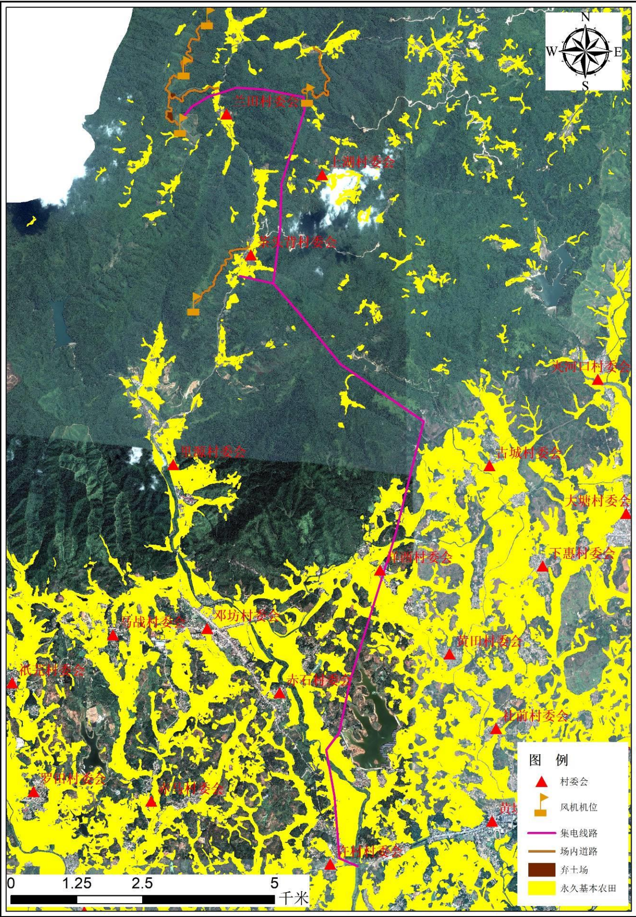
附图 5 项目与基本农田位置关系图
