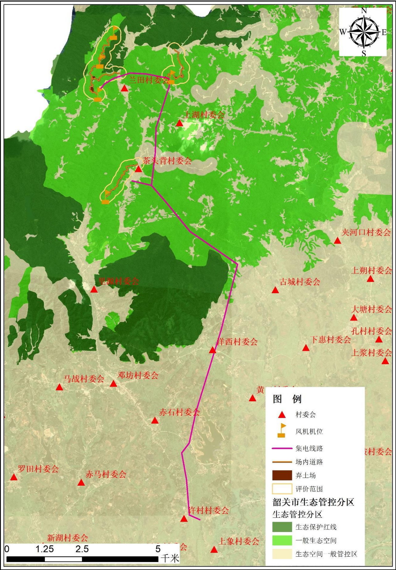
附图 7 项目与韶关市“三线一单”中生态管控分区位置关系图
