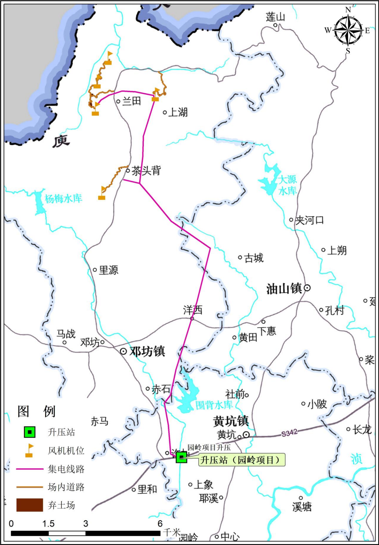
附图 17 项目与园岭项目升压站位置关系图
