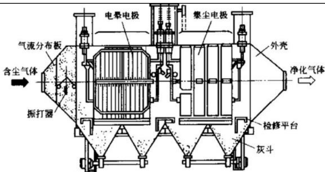
图 4-2 静电除尘工艺原理图
