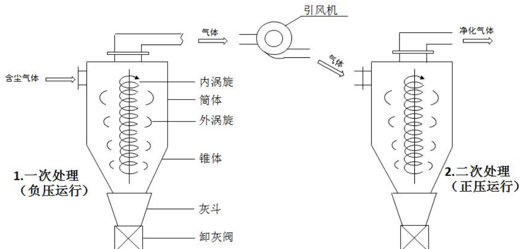
图 4-1 本项目设计旋风分离器工作流程图
