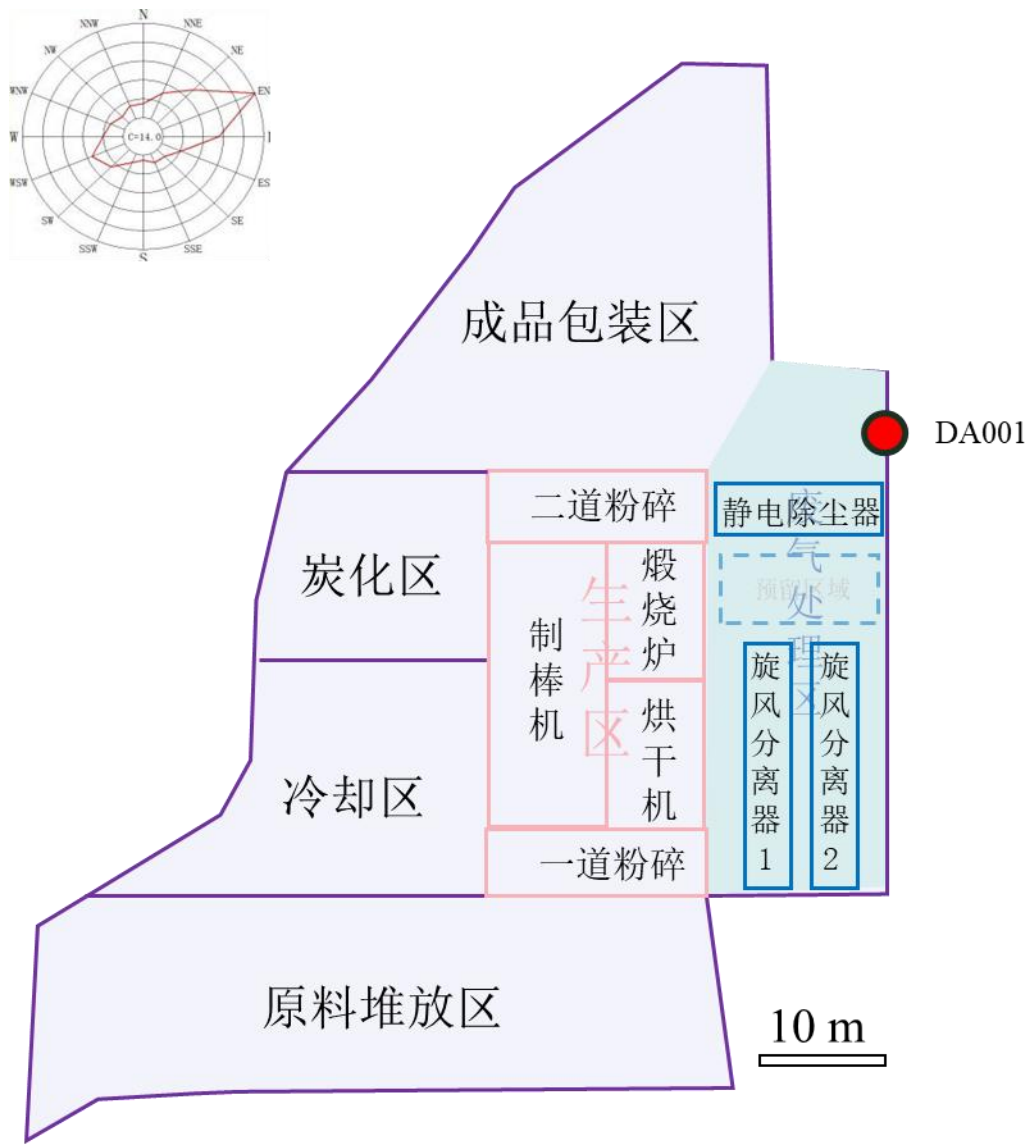
附图 3 本项目平面布置图
