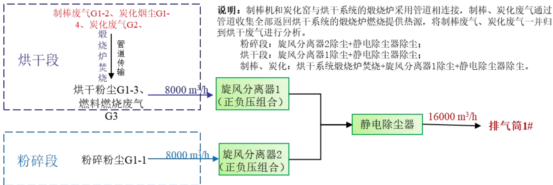
附图 6 本项目废气去向及废气处理设施连接图
