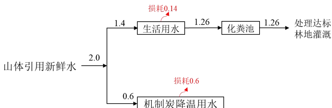
图 2-1 本项目水平衡图（单位：m 3 /d）
