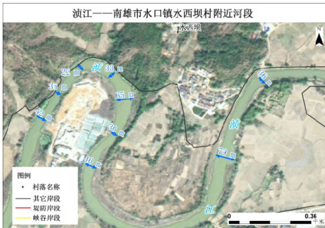
图 6-5 水口镇水西坝村附近河段河势
