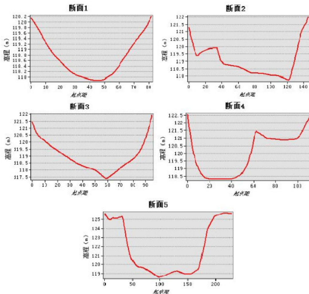
(b) 小水村附近河段断面形态图（右岸-左岸）
