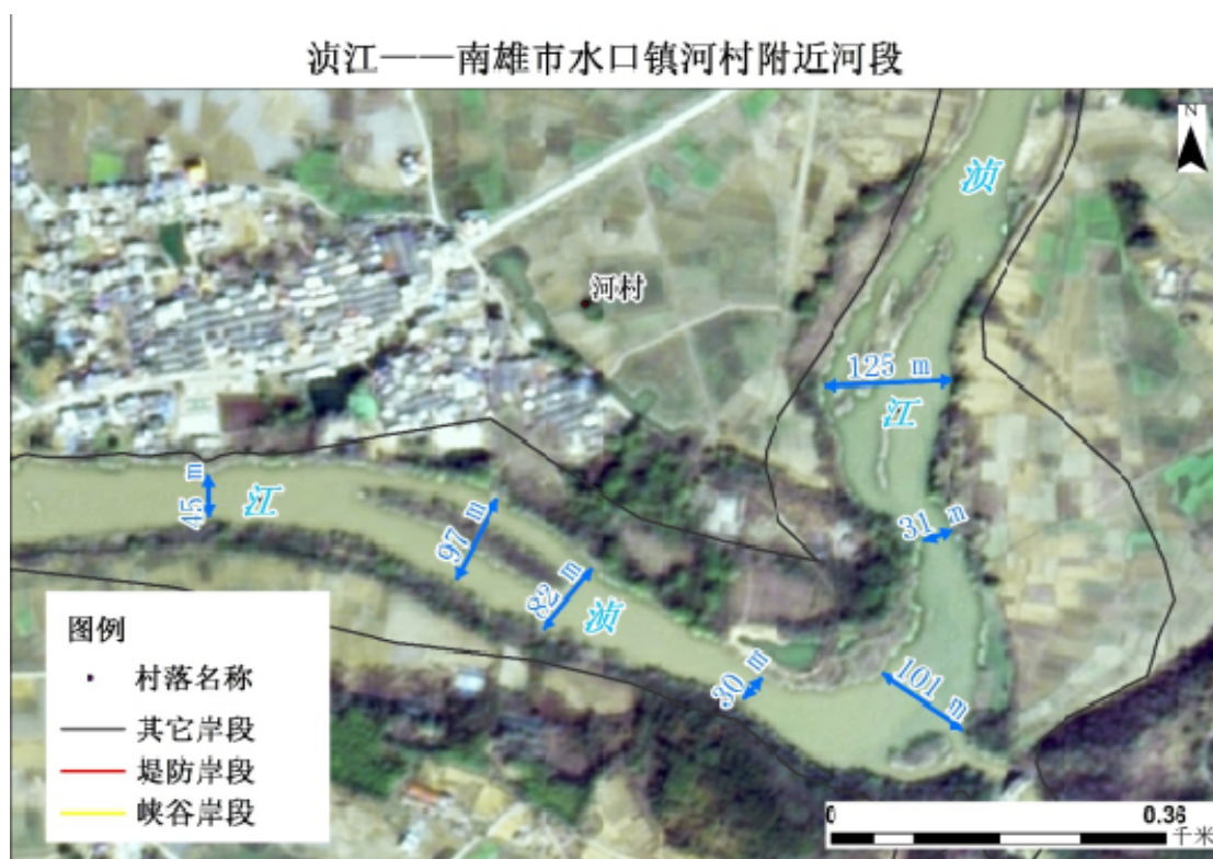
图 6-7 水口镇河村附近河段河势
