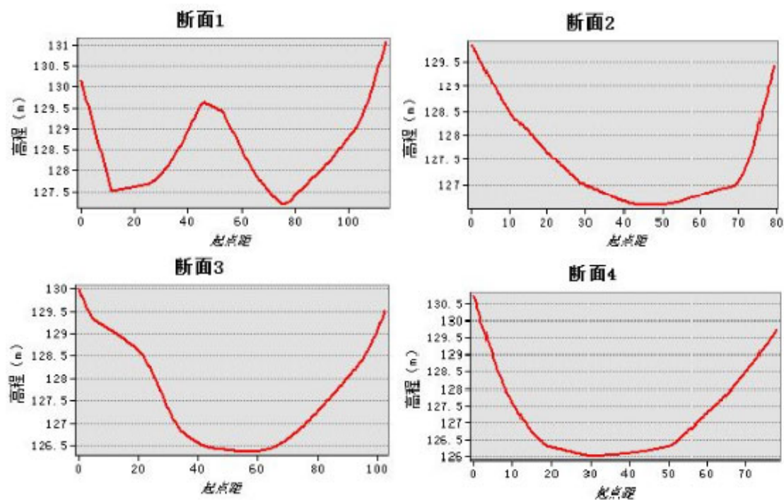
图 6-8 水口镇老李屋村附近河段河势
