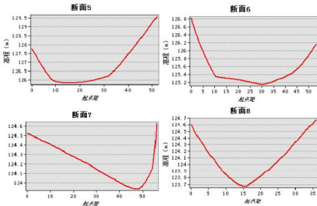
图 6-9 水口镇老李屋村附近河段剖面（右岸-左岸）
