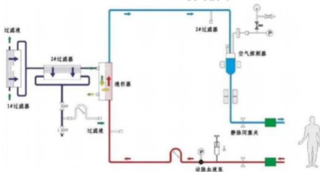
图 3 透析工作原理示意图
