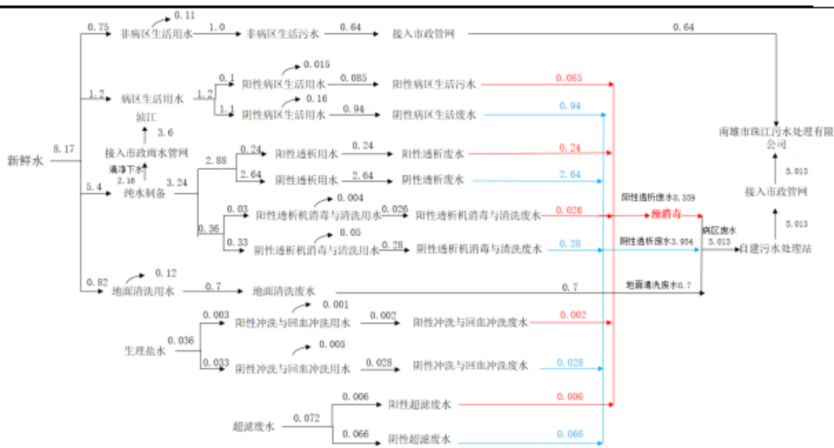
图 4 项目水平衡图 (m 3 /d)
