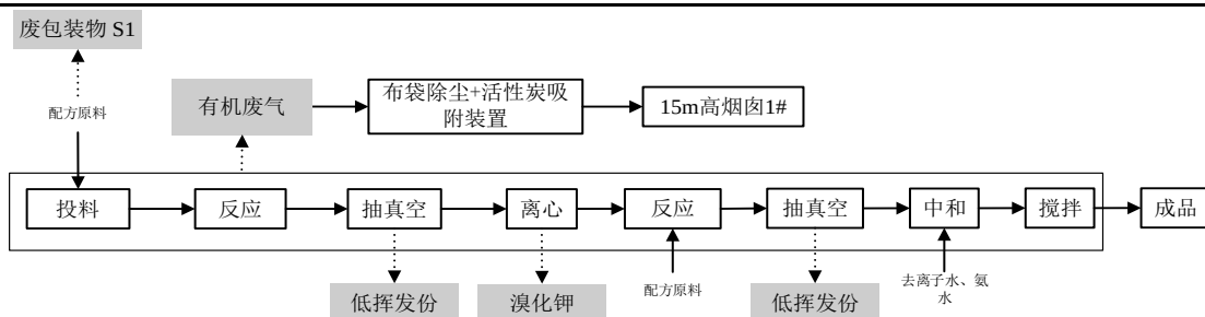
图 13-15 超分散剂生产工艺流程及产污环节图
