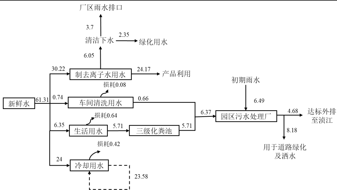
图21 扩建后全厂水平衡图 (m³/d)
