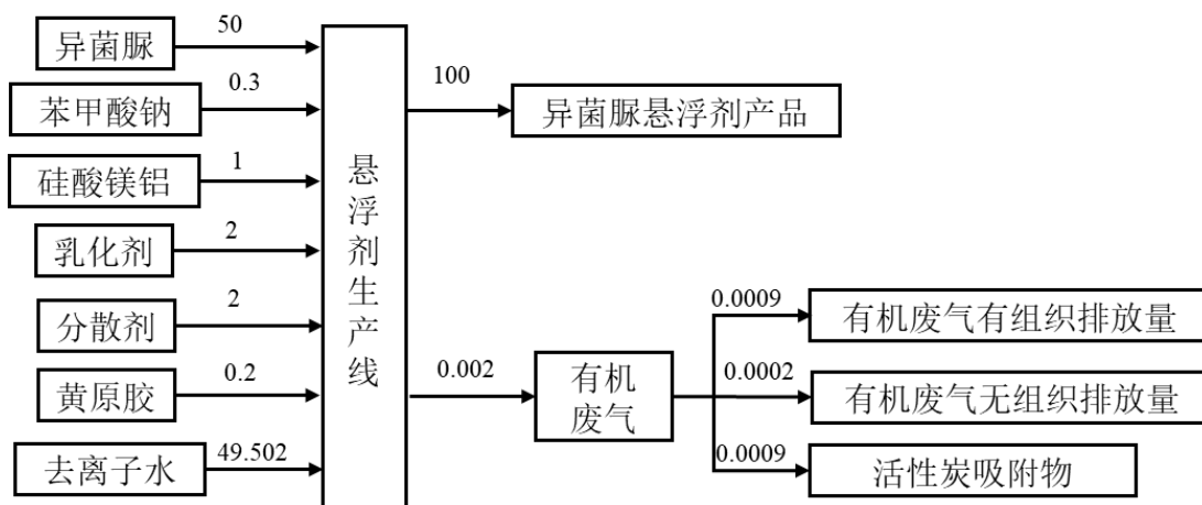
图 1 异菌脲悬浮剂产品物料平衡图 (t/a)
