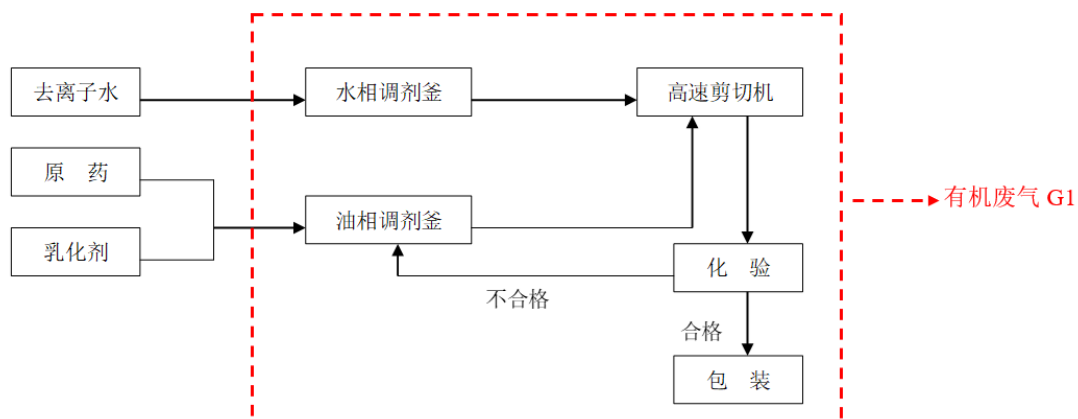
图 9 咪鲜胺水乳剂工艺流程图
