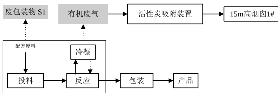
图 13-10 表面处理液生产工艺流程及产污环节图
