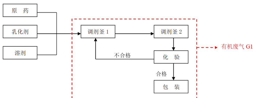
图 12 稻瘟灵乳油工艺流程图
