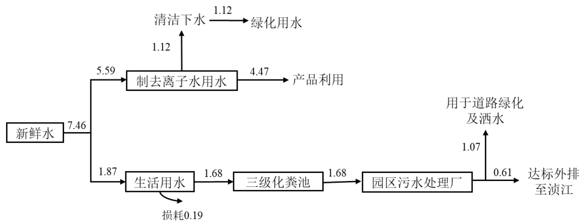
图20 本项目水平衡图 (m 3 /d)
