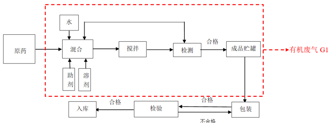
图 10 芸苔素内酯可溶液剂工艺流程图
