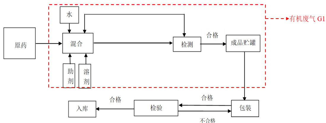
图 11 甲氨基阿维菌素苯甲酸盐微乳剂工艺流程图
