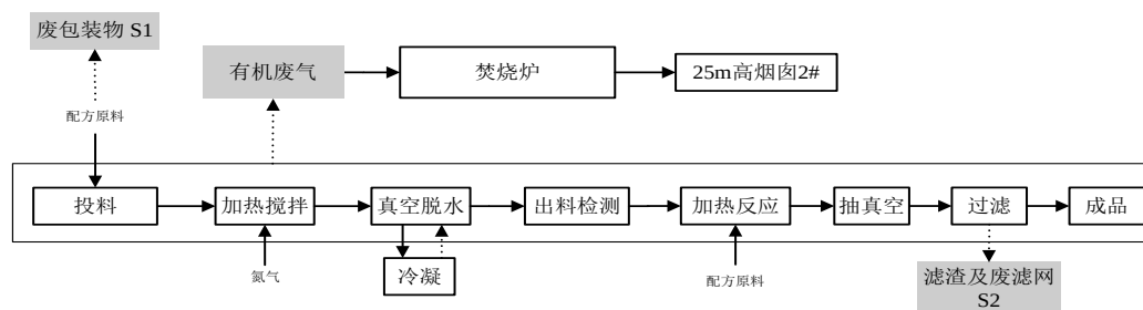
图 13-12 环氧改性丙烯酸树脂生产工艺流程及产污环节图
