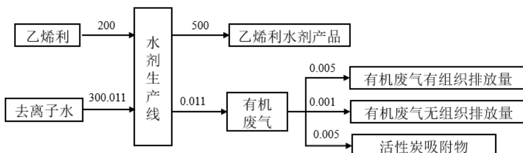
图 2 乙烯利水剂产品物料平衡图 (t/a)
