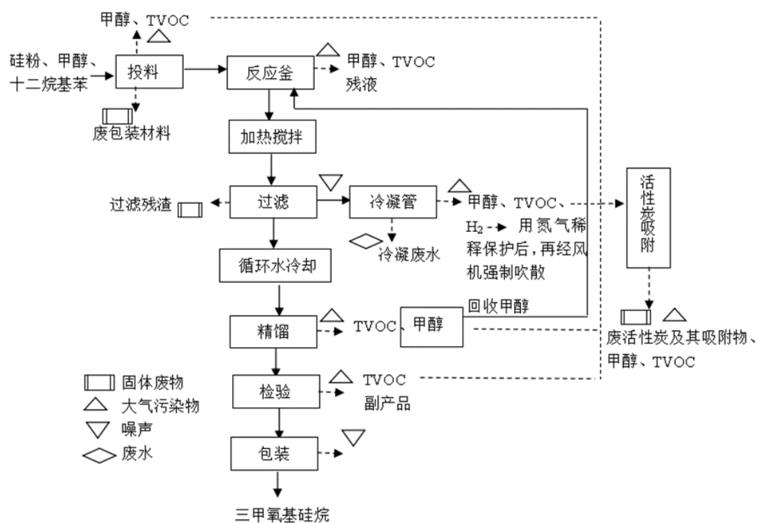
图 13-5 三甲氧基硅烷生产工艺流程及产污环节图
