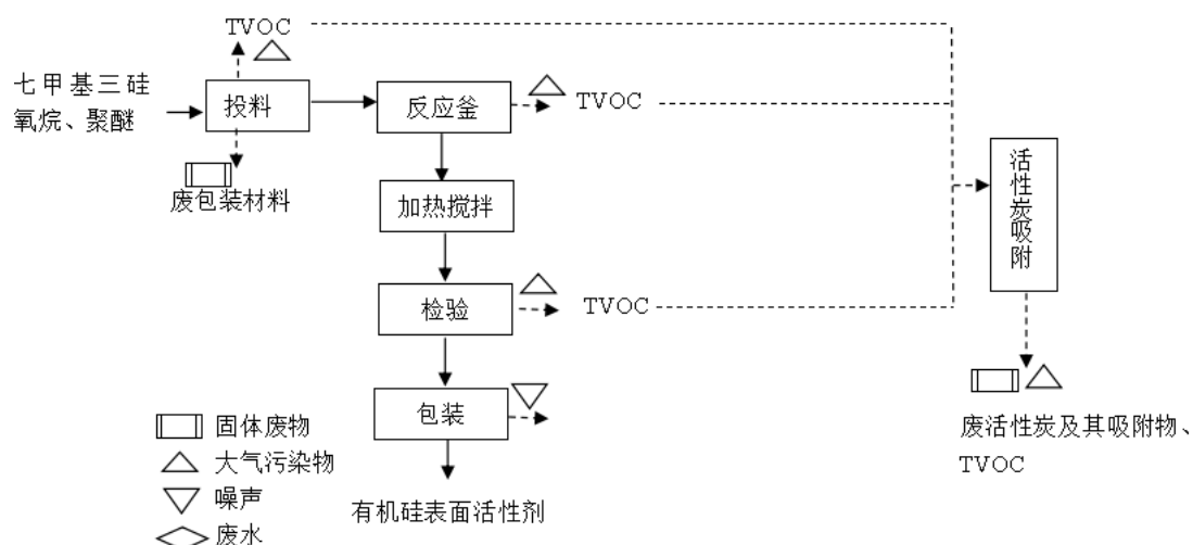
图 13-3 有机硅表面活性剂生产工艺流程及产污环节图
