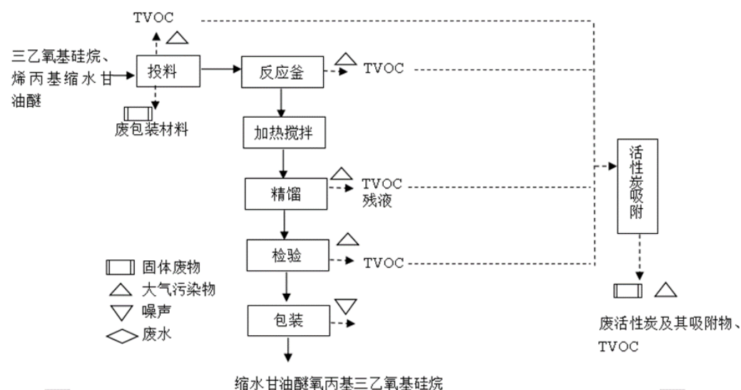
图 13-2 缩水甘油醚丙基三乙氧基硅烷生产工艺流程及产污环节图
