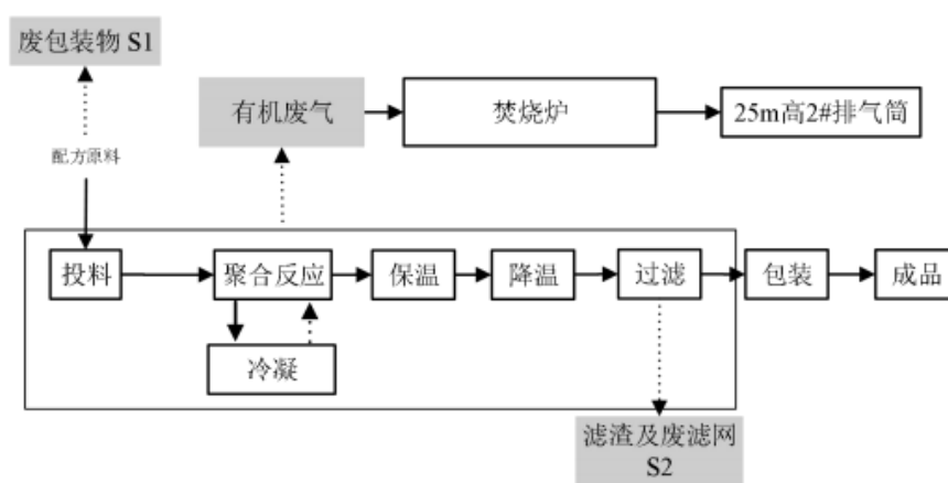
图 13-11 丙烯酸树脂生产工艺流程及产污环节图
