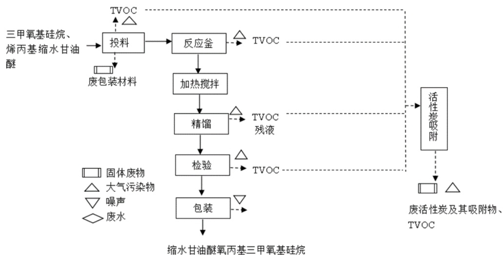
图 13-1 缩水甘油醚氧丙基三甲氧基硅烷生产工艺流程及产污环节图
