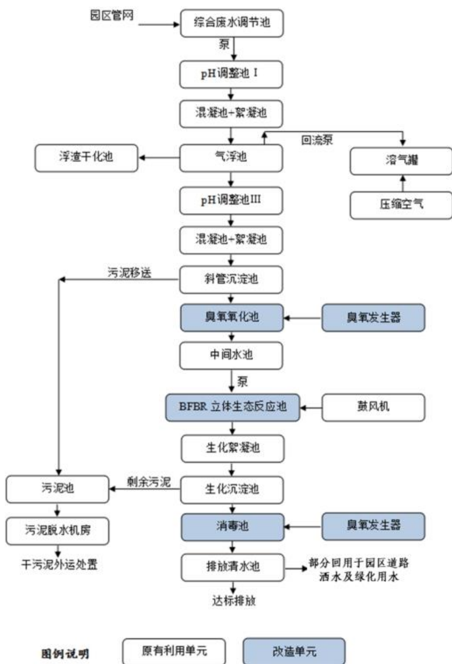
图22 园区污水处理厂废水处理工艺流程图
