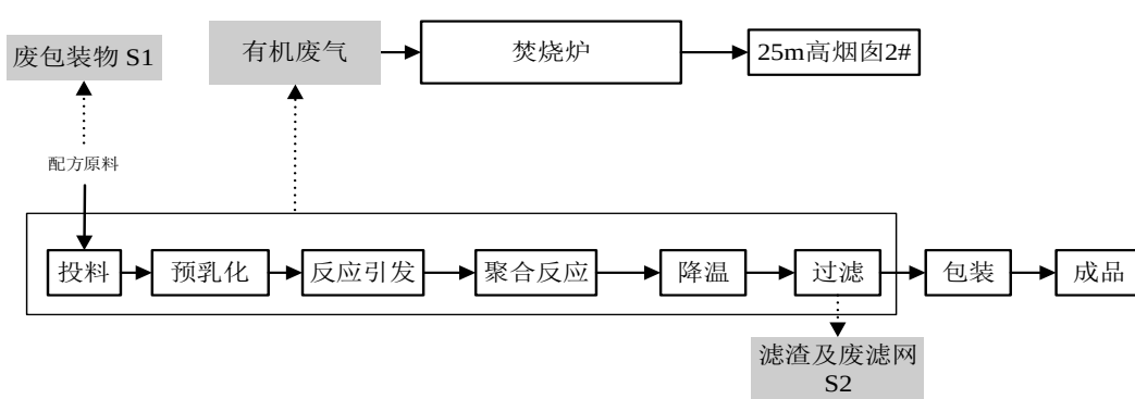
图 13-18 水性有机硅改性丙烯酸乳液粘合剂生产工艺流程及产污环节图
