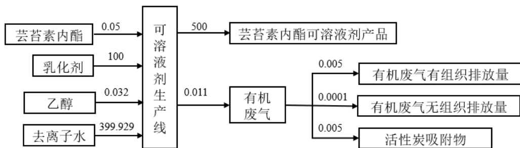
图 5 芸苔素内酯可溶液剂产品物料平衡图 (t/a)
