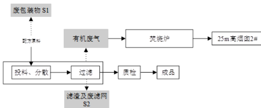
图 13-19 木蜡油（水性）生产工艺流程及产污环节图
