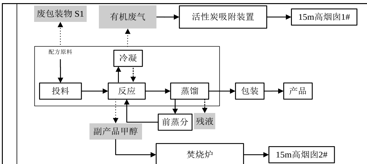
图 13-9 乙烯基硅烷生产工艺流程及产污环节图
