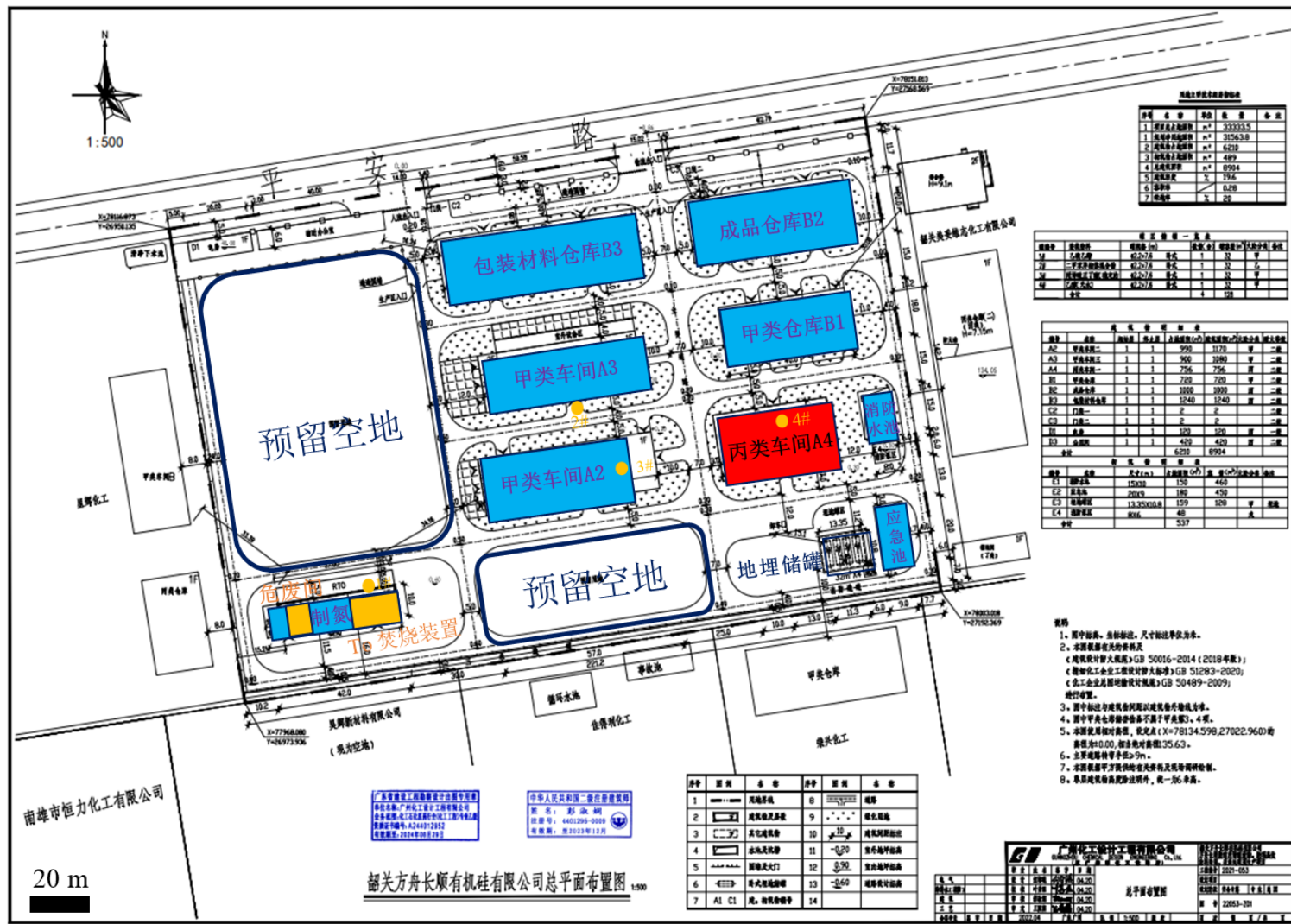
附图 5 厂区总平面布置图
