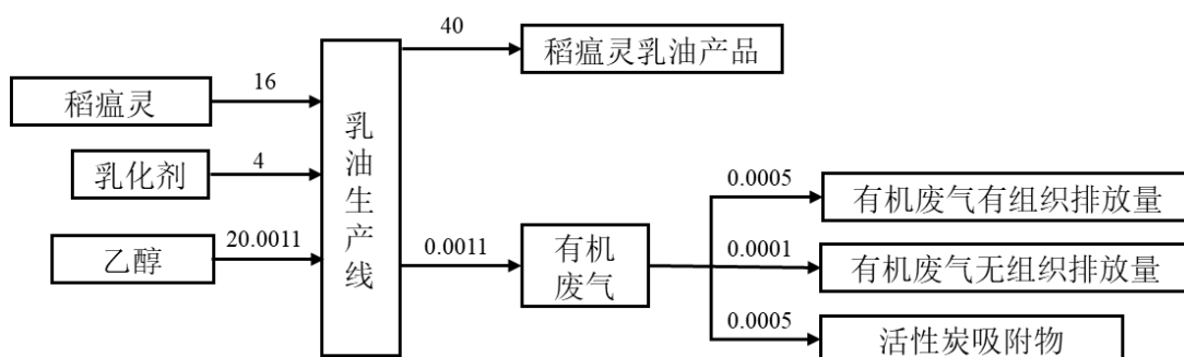
图 6 稻瘟灵乳油产品物料平衡图 (t/a)
