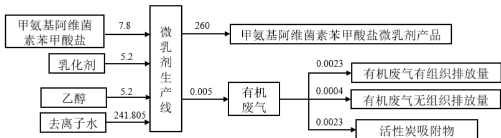
图 4 甲氨基阿维菌素苯甲酸盐微乳剂产品物料平衡图 (t/a) (5) 芸苔素内酯可溶液剂
