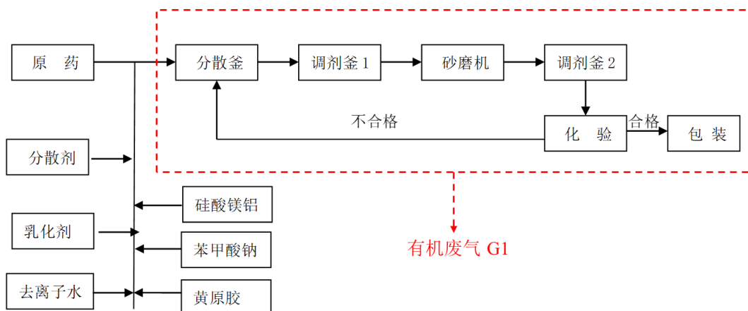
图7 异菌脲悬浮剂工艺流程图
