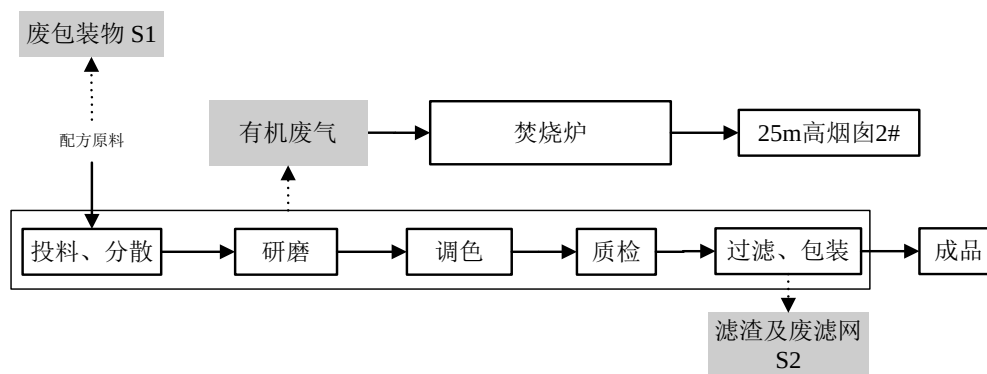
图 13-17 UV 光固化涂料生产工艺流程及产污环节图
