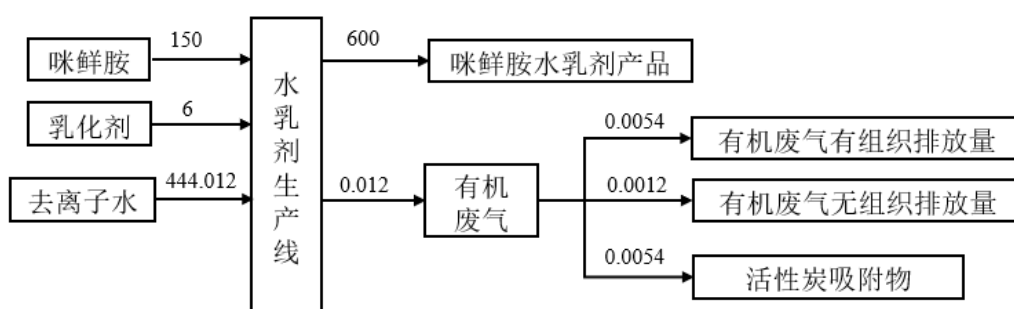
图 3 咪鲜胺水乳剂产品物料平衡图 (t/a)
