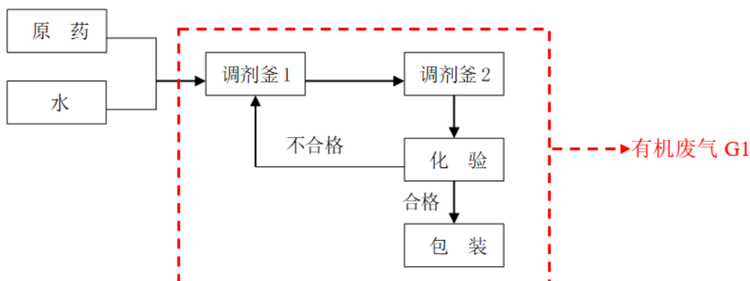
图8 乙烯利水剂工艺流程图
