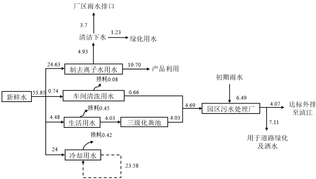
图 14 全厂现有项目水平衡图（单位：m³/d）
