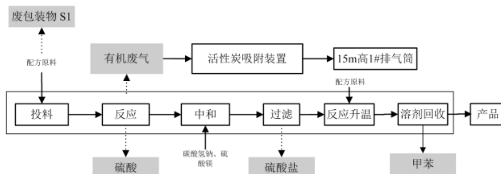
图 13-14 有机硅涂料助剂生产工艺流程及产污环节图
