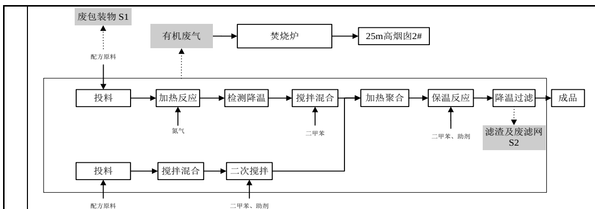
图 13-13 醇酸改性丙烯酸树脂生产工艺流程及产污环节图
